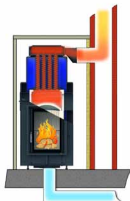
Tryb kotła z podłączeniem bezpośrednim
